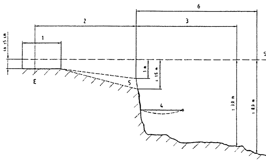
Рисунок 1. Зоны посадки на кресельных КД
