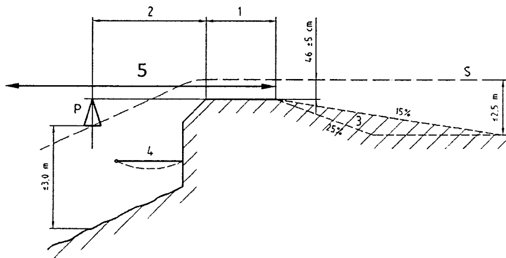
Рисунок 2. Зоны высадки кресельных канатных дорог
